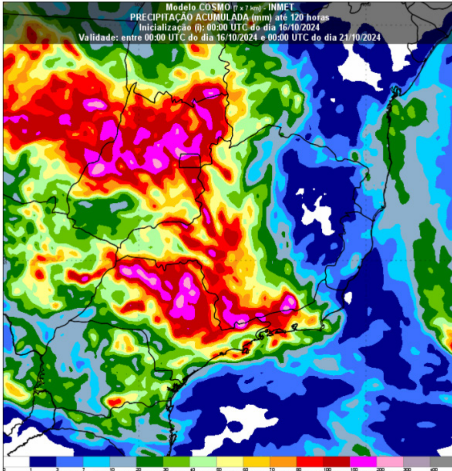
Figura 1 – Simulação do modelo COSMO/INMET para o acumulado de chuva dos próximos dias. Mapa com previsão meteorológica para o estado de São Paulo até dia 21/10
